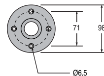
Fot, ingår i golv/väggfäste
