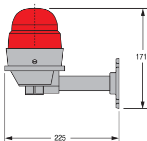
Enkelt hinderljus, väggfäste Vikt 1,6 kg
