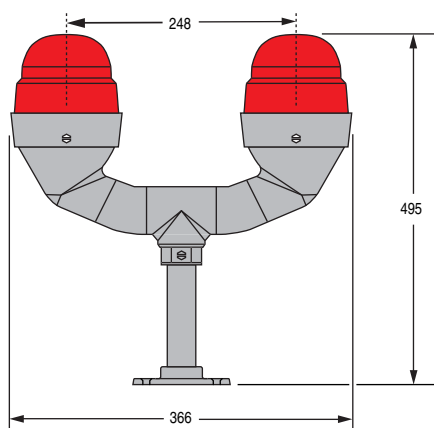
Dubbelt hinderljus, golvfäste Vikt 2,8 kg
