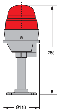
Enkelt hinderljus, golvfäste Vikt 1,6 kg
