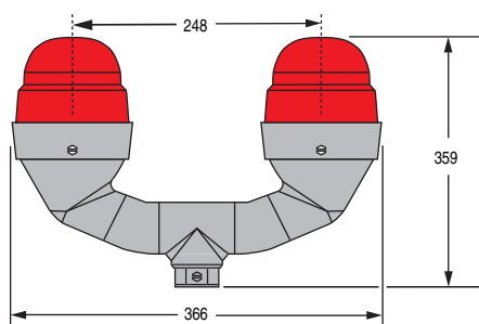
Dubbelt hinderljus Vikt 2,1 kg
